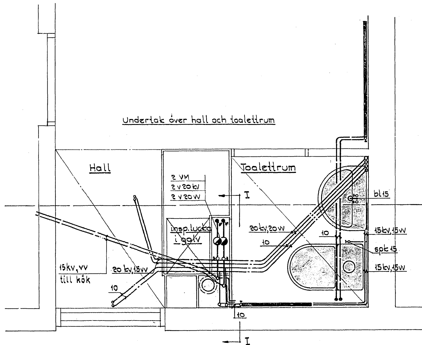
Plan Skala 1:20
